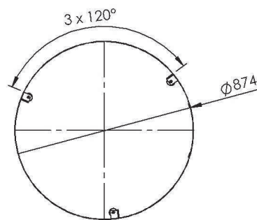
COUPE A-A
